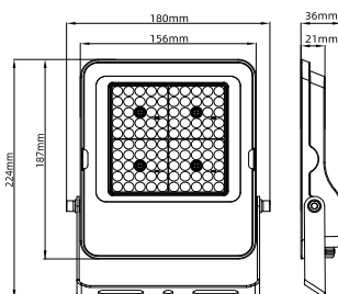
05 ZGSM-FL12-200
