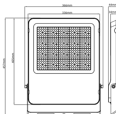
06 ZGSM-FL12-240 / 300
