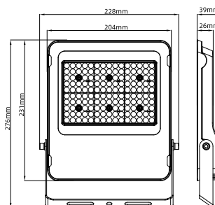
06 ZGSM-FL12-240 / 300
