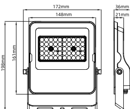
04 ZGSM-FL12-150
