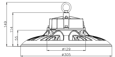
04 ZGSM-HB12-200W/240W □
